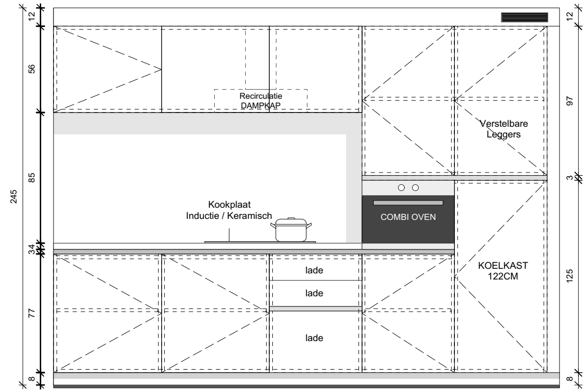
AANZICHT - KEUKEN
